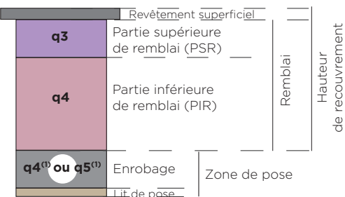
COUPE TROTTOIR
