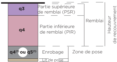
COUPE ACCOTEMENT
